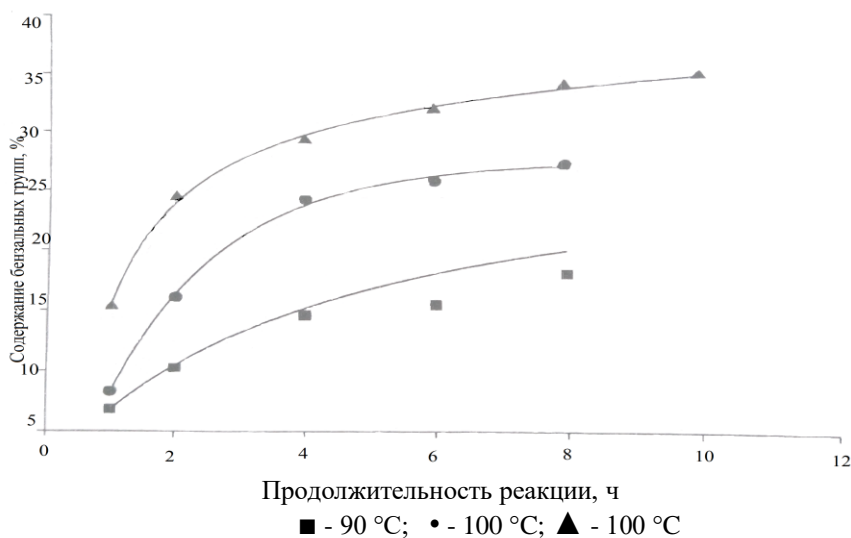
Рисунок 5 - Содержание бензильных групп при различных температурах
